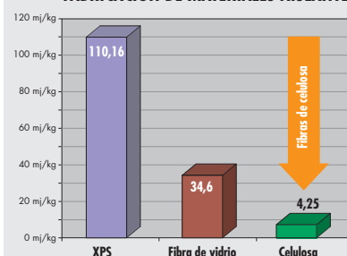
ENERGÍA PRIMARIA NECESARIA PARA LA FABRICACIÓN DE MATERIALES AISLANTES
